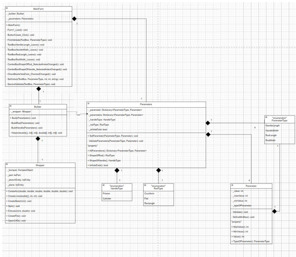
Рисунок 7.2 – UML диаграмма классов после реализации плагина «Отвёртка»
